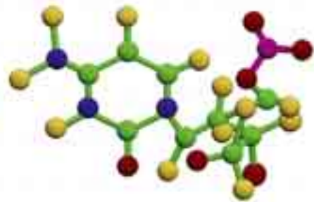
Cytosine
